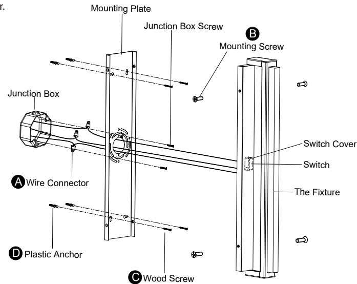
Fig. 2 Wiring
