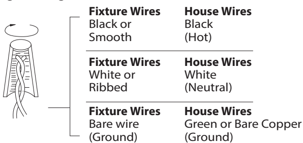
Fig. 2 Wiring
