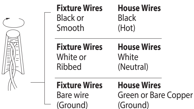
Fig. 2 Wiring
